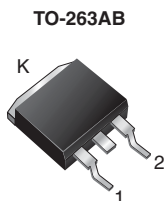
TO-263AB
