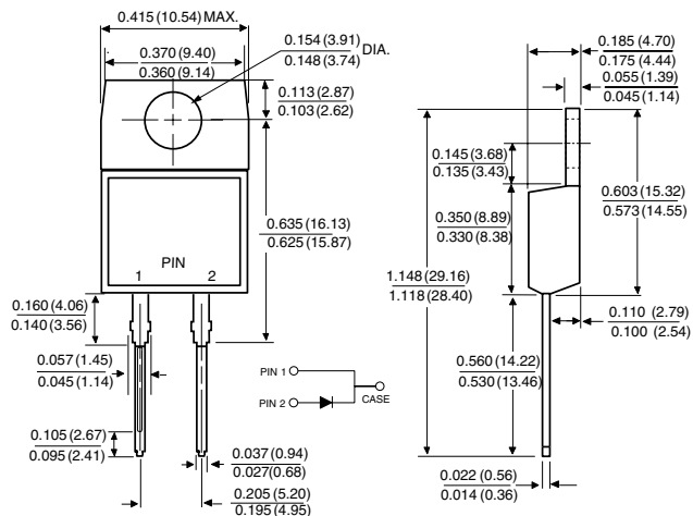
TO-220AC
