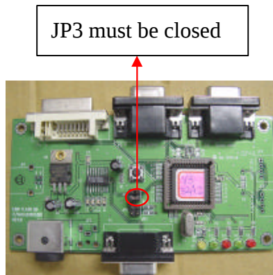
V3 Fixture
