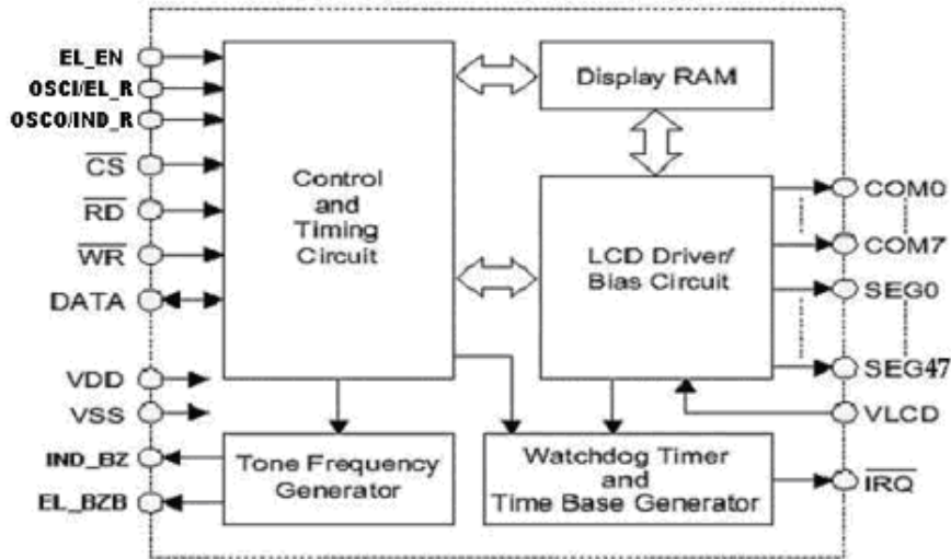
方块图
