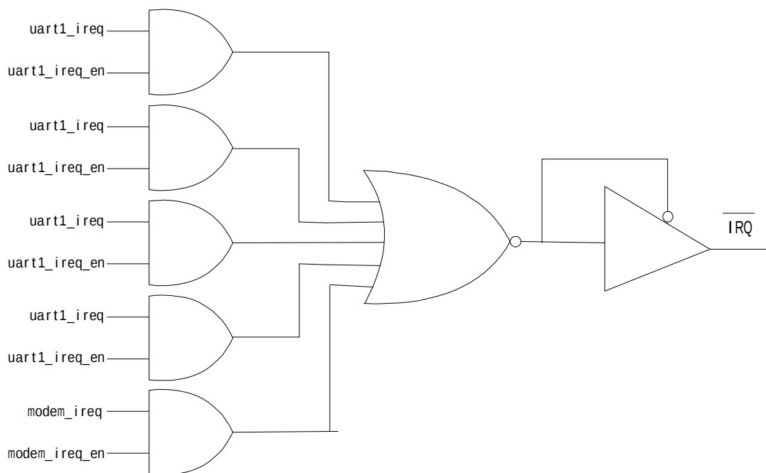
图 8.3 VK3232 中断结构图
