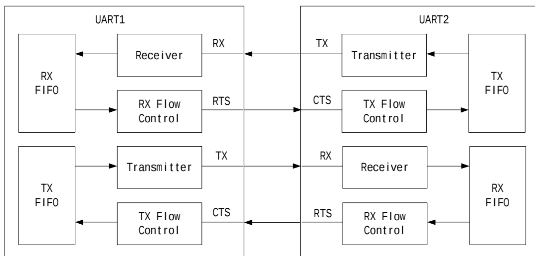
图 11.3.3.1 硬件流量控制示意图
