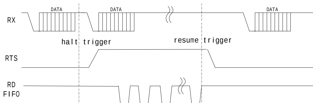
图 11.3.3.2 硬件流量操作时序图
