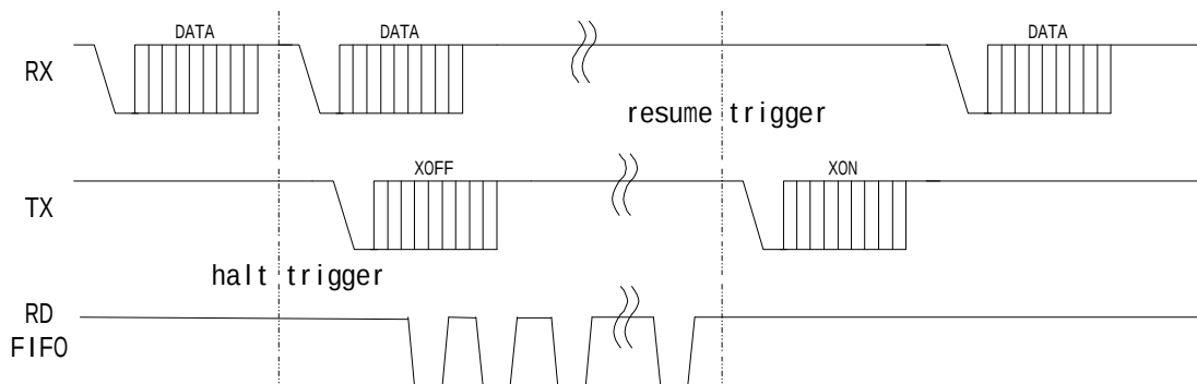
图 11.3.2 XON/XOFF 发送操作
