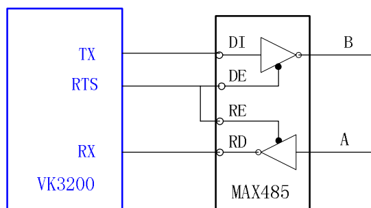
图 11.5.1 RS485 连接图
