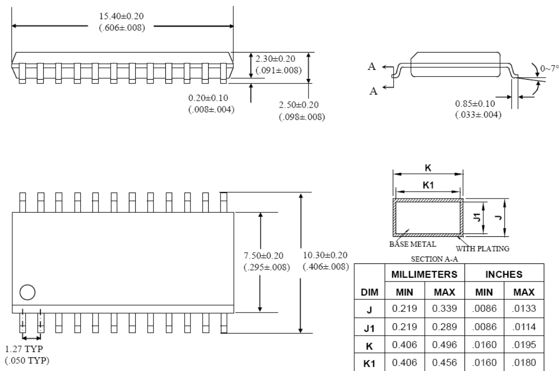
图 13.1 SOP24 封装信息
