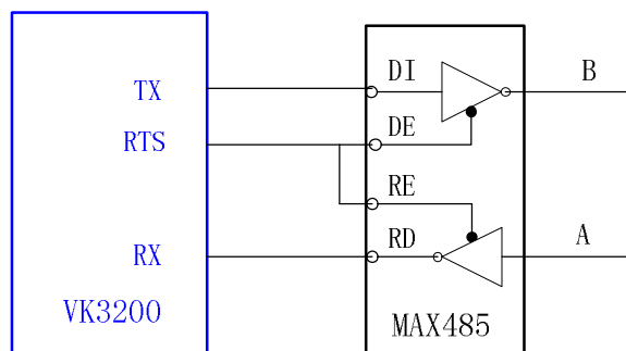
图 11.4.1 RS485 连接图
