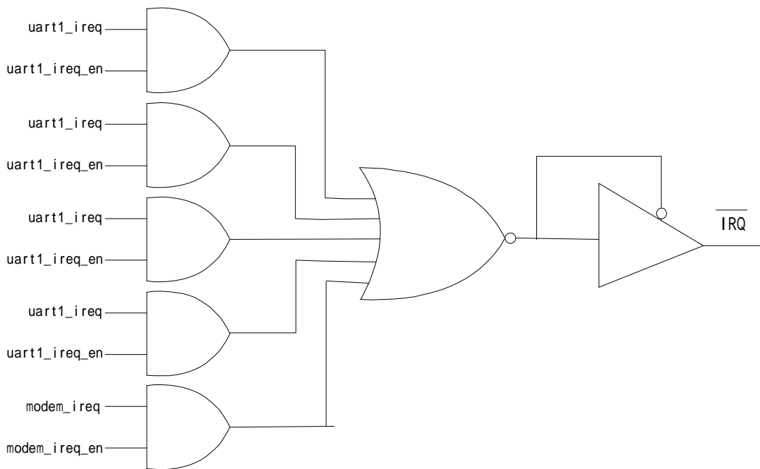
图 8.3 VK3266 中断结构图
