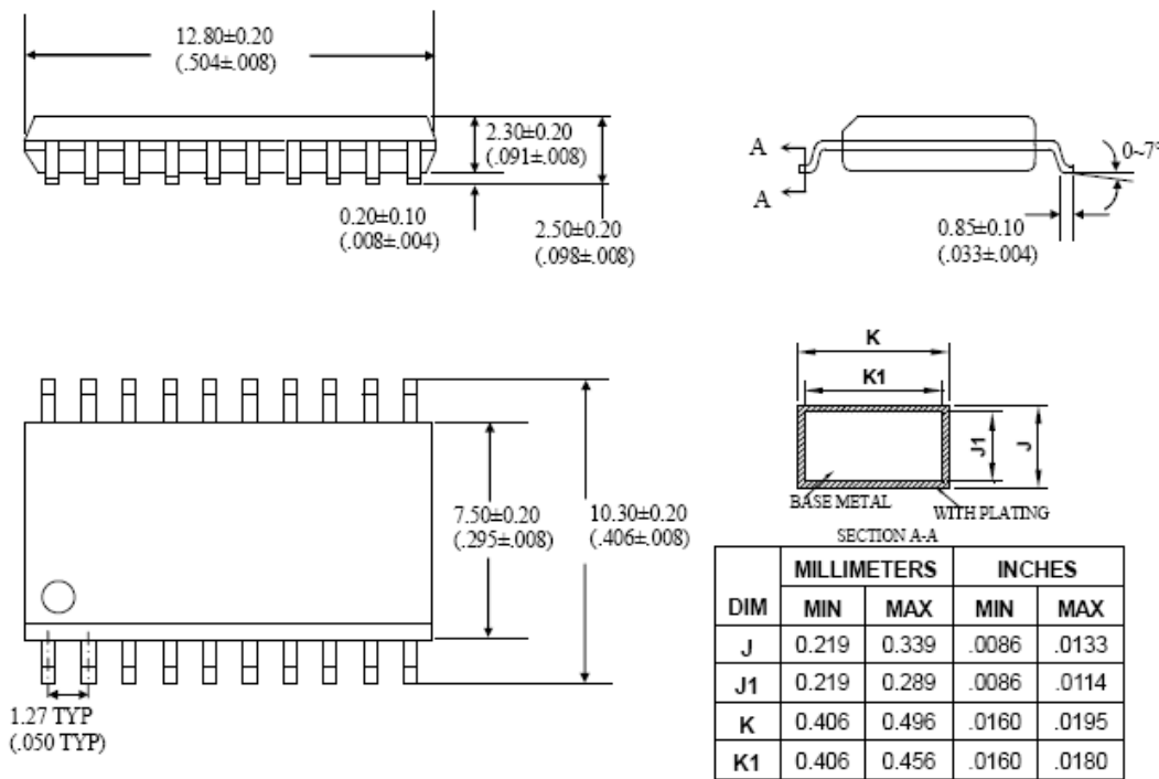
图15.1 SOP20封装信息
