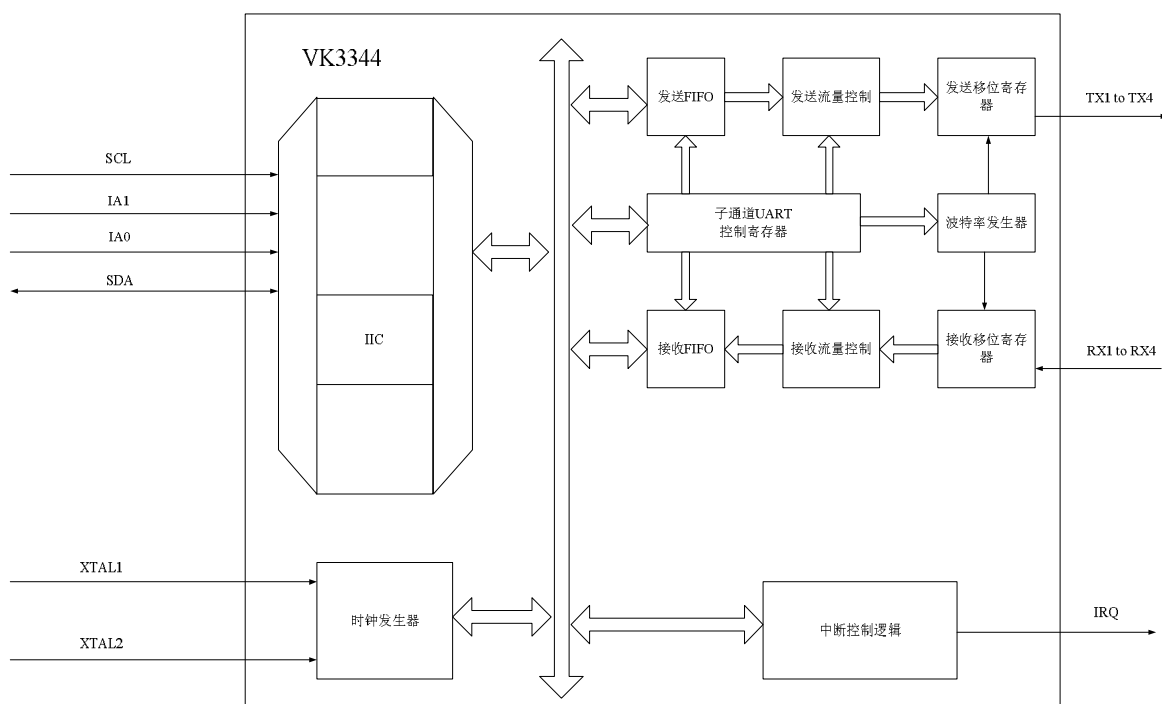
图5.1 VK3344 原理框图
