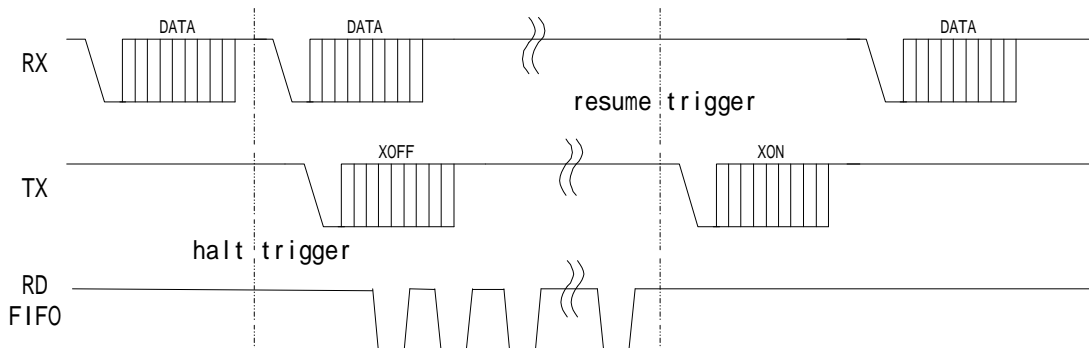
图 13.3.2 XON/XOFF 发送操作
