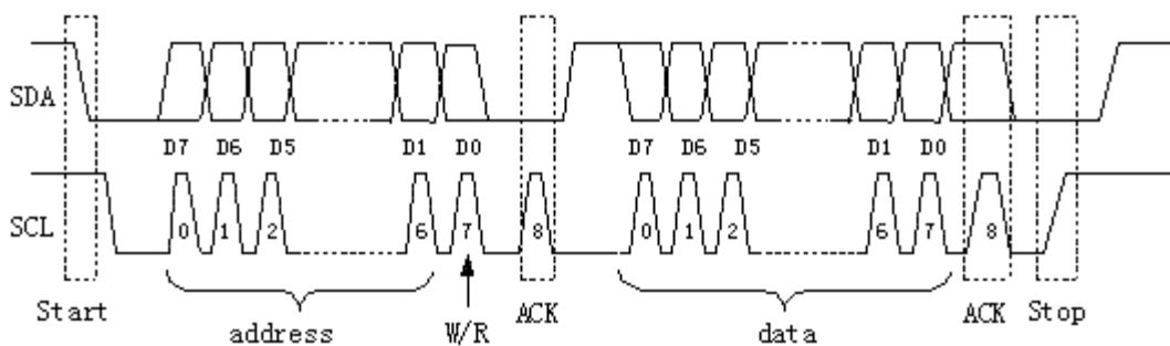
图 12.1.3 IIC 传输协议和格式
