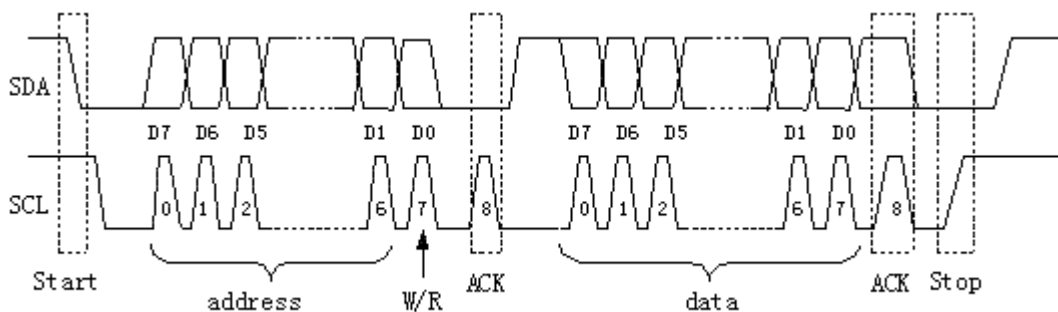
图 12.1.3 IIC 传输协议和格式
