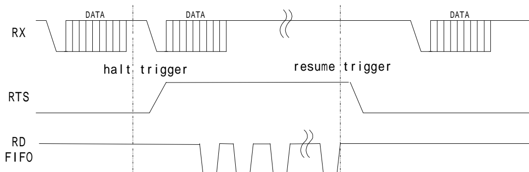
图 13.3.3.2 硬件流量操作时序图
