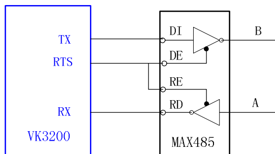
图 13.5.1 RS485 连接图
