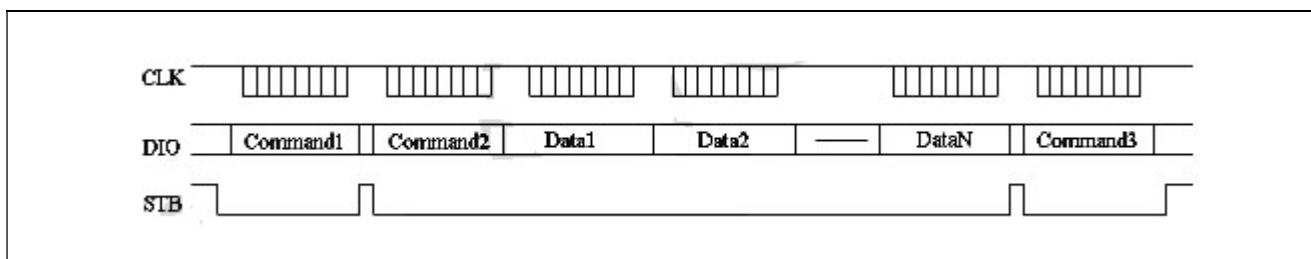
图 2. 地址增加模式的串行数据传输
