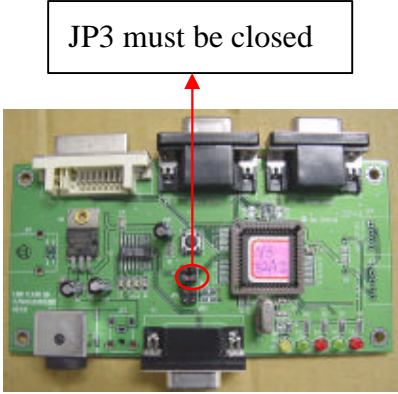
V3 Fixture
