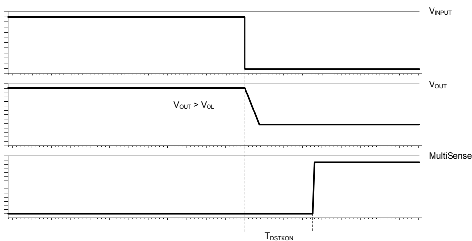
Figure 8. T_{DSTKON}
