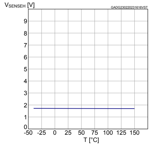
Figure 31. V_{senseh} vs. T_{case}
