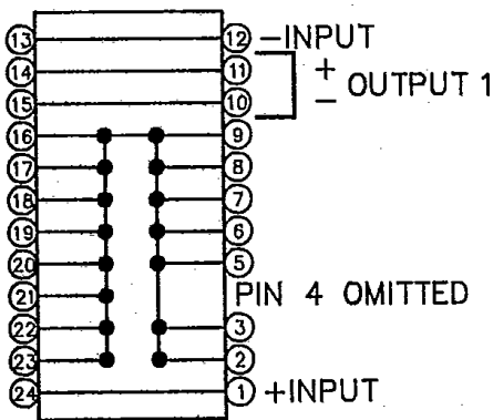
TOP VIEW VA
