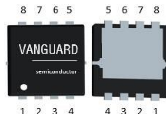
PDFN3333
