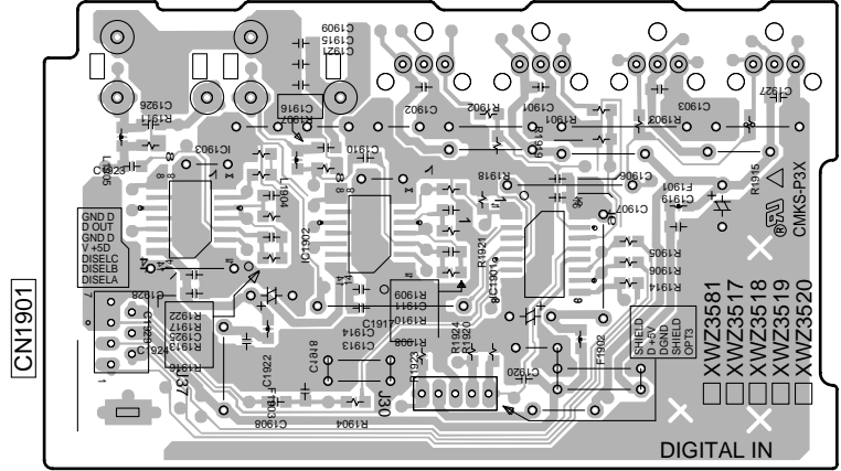
CN1902 (XNP3052-C) IC1903 IC1902 IC1901
