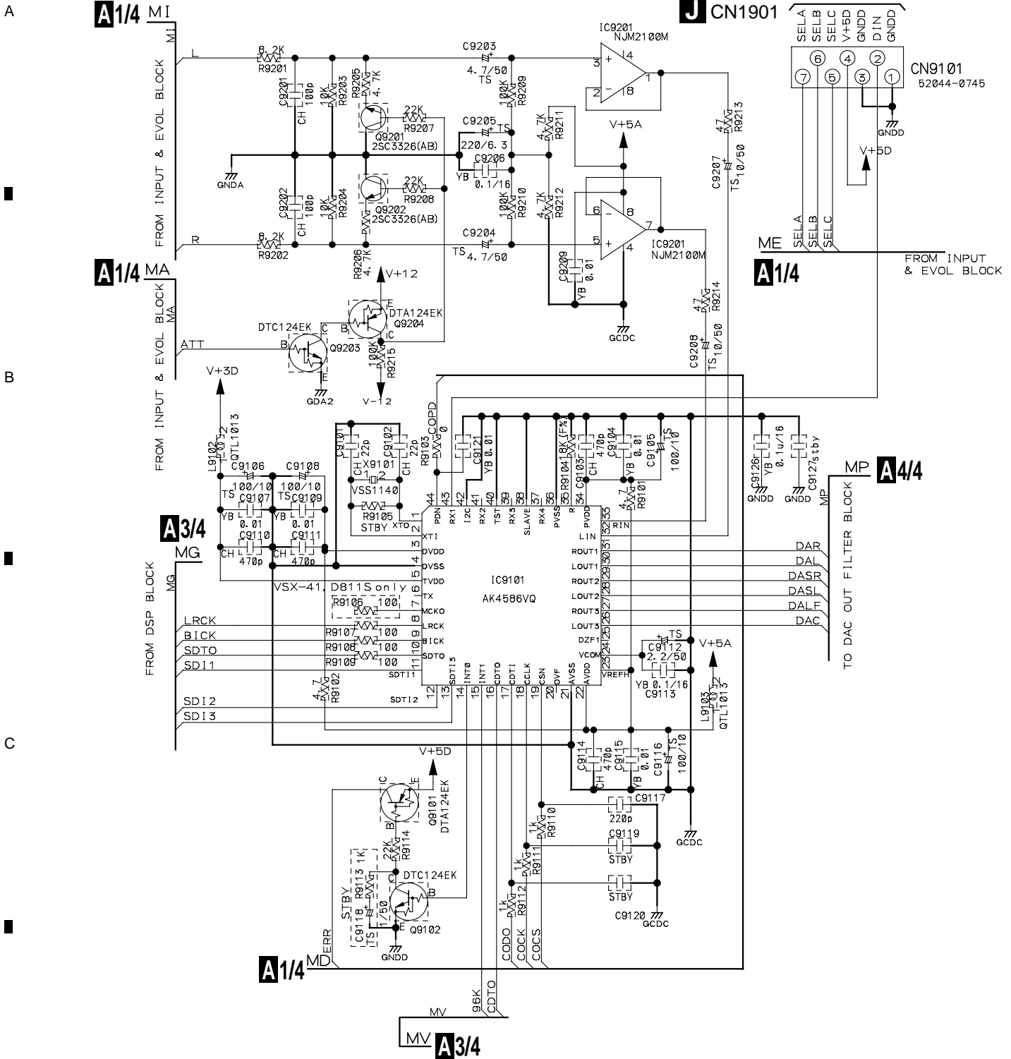
A 2/4 D.D & INPUT ASSY (XWX3047)
