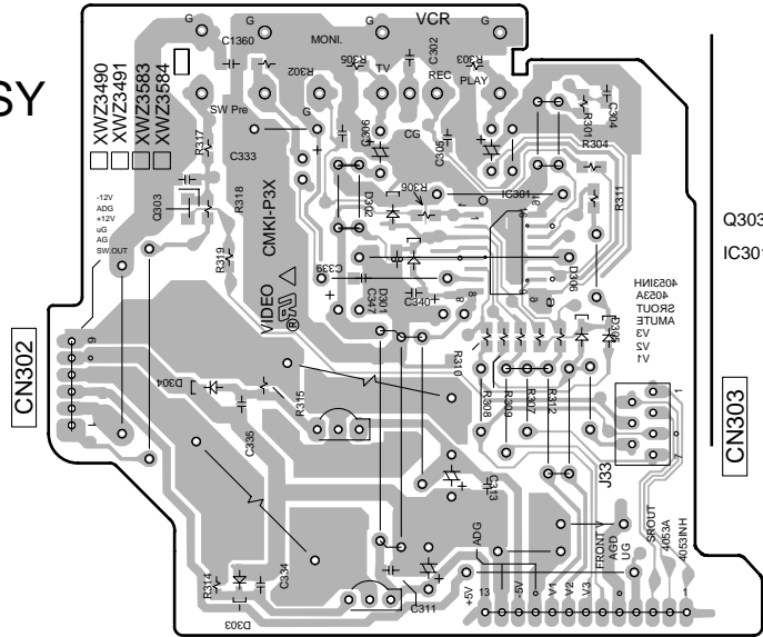
(XNP3052-C) CN301
