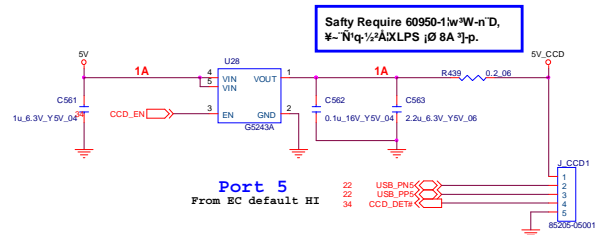
CCD
