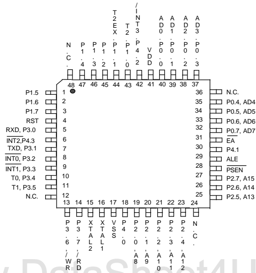
48-Pin LQFP (W78E62BD)
