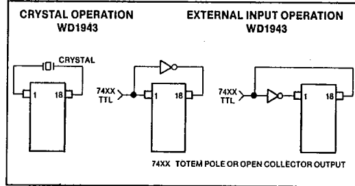
CRYSTAL/CLOCK OPTIONS
