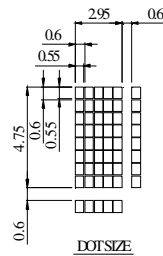
DOTSIZE
