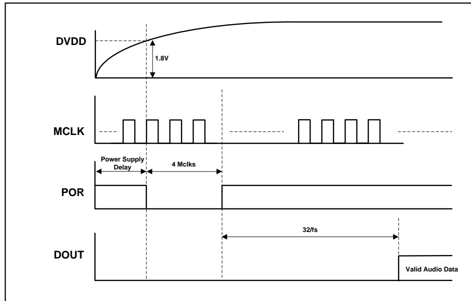
Figure 5 POR Timing
