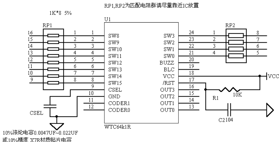
图 4: WTC64K1R 应用原理图
