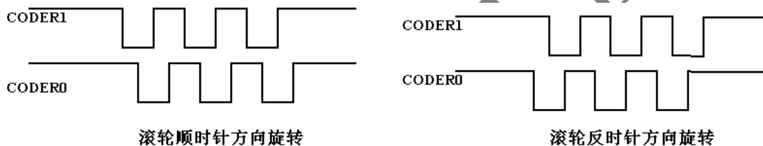
图 3:触摸滚轮输出时序图
