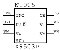
X9503P N????
