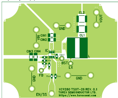
Top Layer (1)
