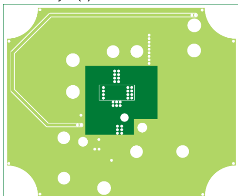
Bottom Layer (4)
