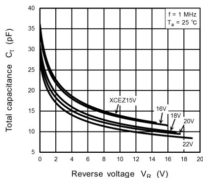
Fig. 11.1.7 C_t - V_R (3)
