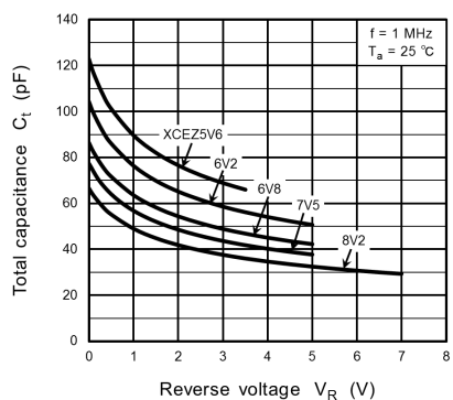
Fig. 11.1.5 C_t - V_R (1)
