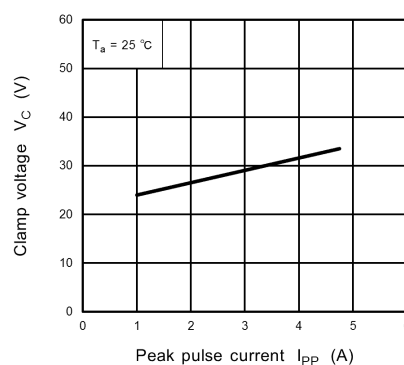
Fig. 11.16.2 V_C - I_{PP}
