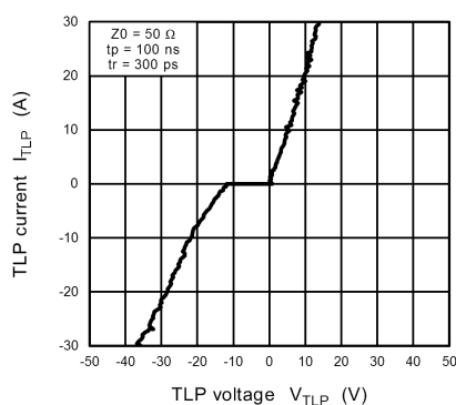
Fig. 11.10.1 I_{TLP} - V_{TLP}
