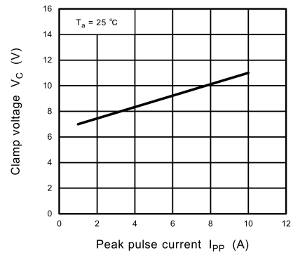
Fig. 11.4.2 V_C - I_{PP}
