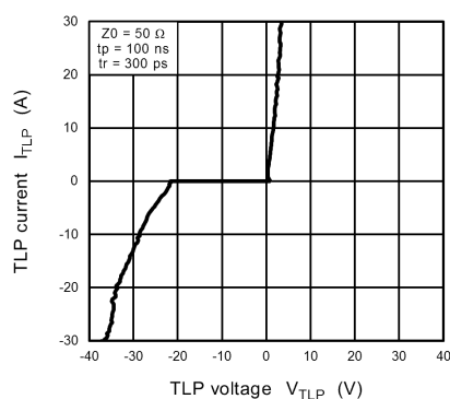
Fig. 11.16.1 I_{TLP} - V_{TLP}
