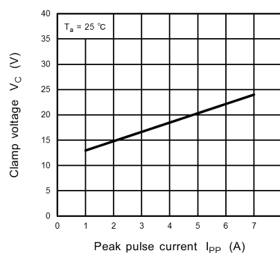
Fig. 11.10.2 V_C - I_{PP}
