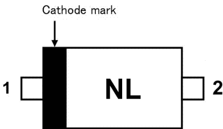
Fig. 9.1 XCEZ5V6
