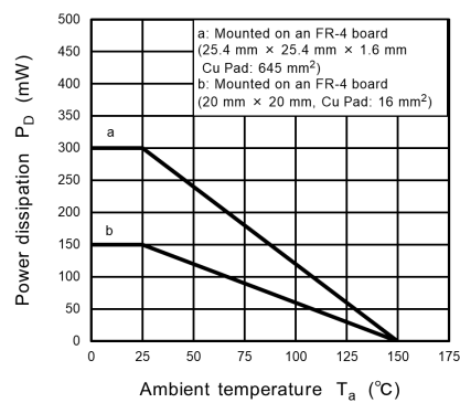
Fig. 11.1.10 P_D - T_a
