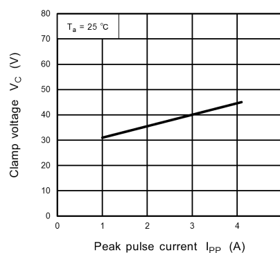
Fig. 11.18.2 V_C - I_{PP}
