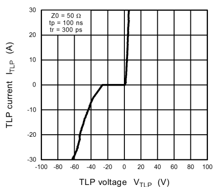
Fig. 11.18.1 I_{TLP} - V_{TLP}
