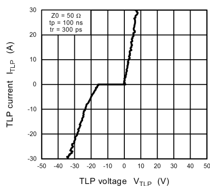
Fig. 11.13.1 I_{TLP} - V_{TLP}
