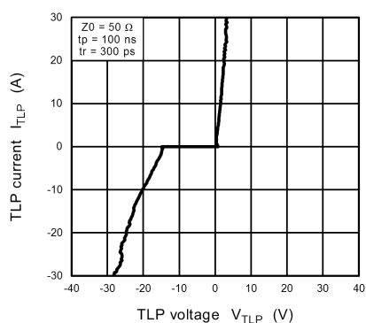
Fig. 11.12.1 I_{TLP} - V_{TLP}
