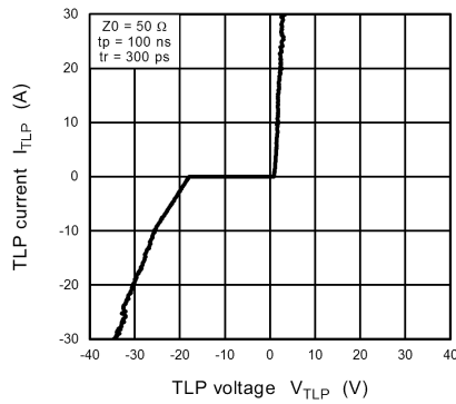
Fig. 11.14.1 I_{TLP} - V_{TLP}
