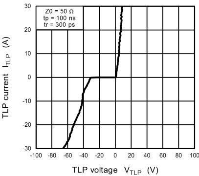
Fig. 11.19.1 I_{TLP} - V_{TLP}
