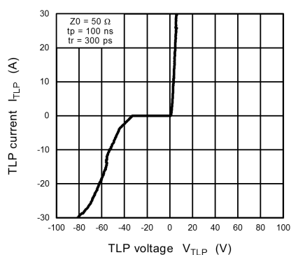
Fig. 11.20.1 I_{TLP} - V_{TLP}
