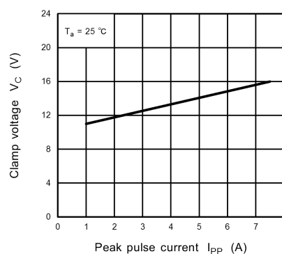
Fig. 11.8.2 V_C - I_{PP}
