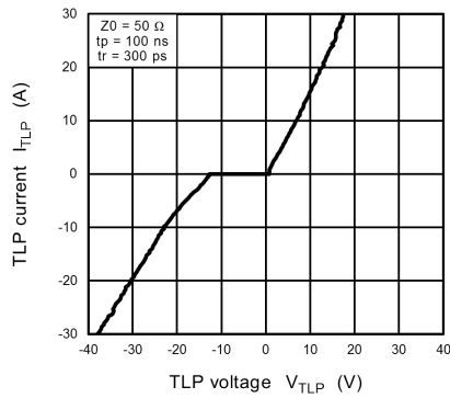
Fig. 11.11.1 I_{TLP} - V_{TLP}
