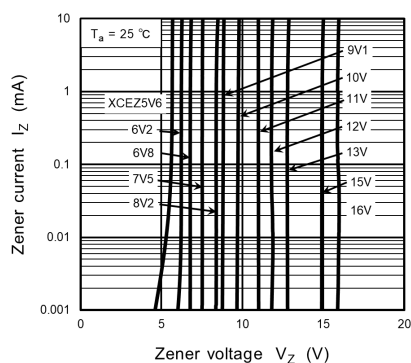
Fig. 11.1.1 I_Z - V_Z(1)
