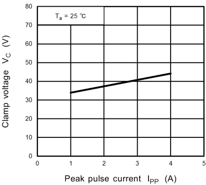
Fig. 11.19.2 V_C - I_{PP}
