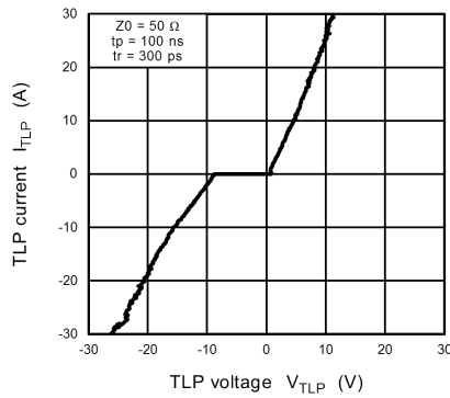
Fig. 11.7.1 I_{TLP} - V_{TLP}
