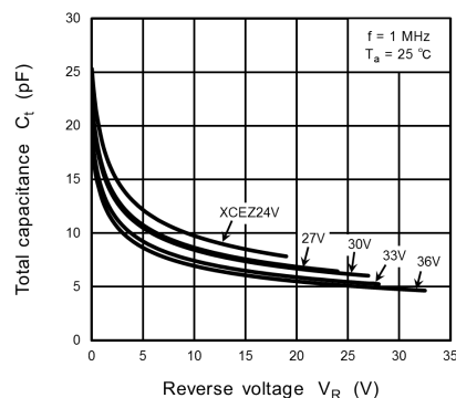
Fig. 11.1.8 C_t - V_R (4)
