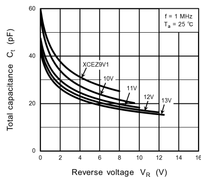
Fig. 11.1.6 C_t - V_R (2)
