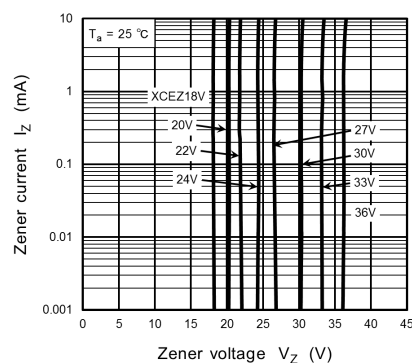
Fig. 11.1.2 I_Z - V_Z(2)
