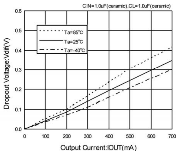
XC6210 (VOUT:5.0V)
