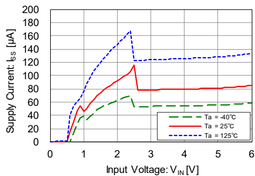
XD6239x251
