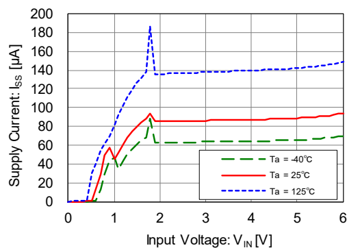
XD6239x181
