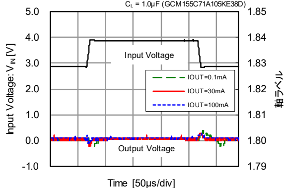
XD6239x181
