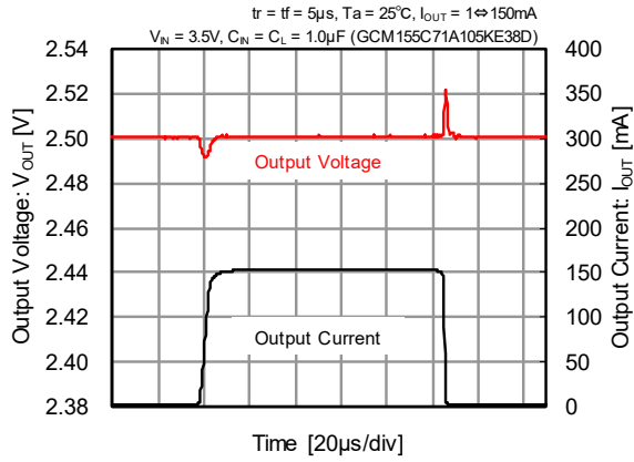
XD6239x251
