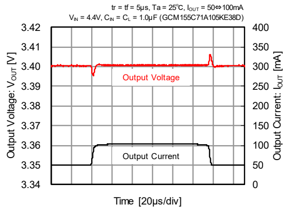
XD6239x341
