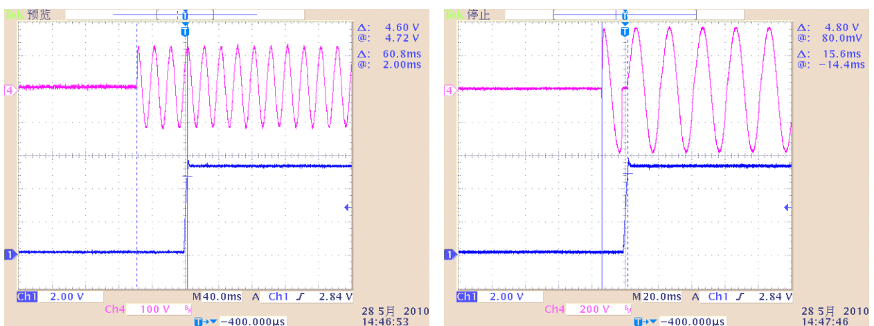
图3 90V 启动延时波形
