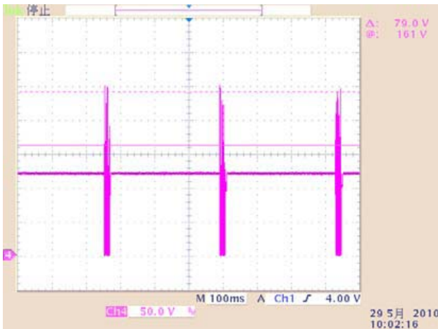
图 11 85V Voc 波形 输出短路
