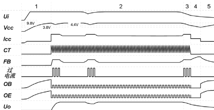
图 2 全局波形示意图
