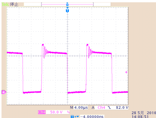
图 7 85V Voc 波形 I_o=0.5A
