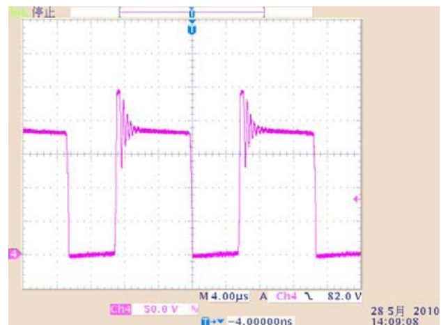
图 8 85V Voc 波形 I_o=1A
