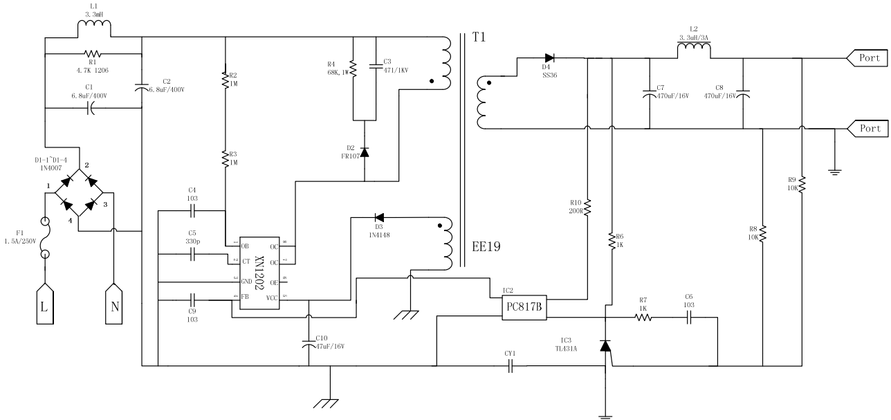
5V1A 反激式开关电源
