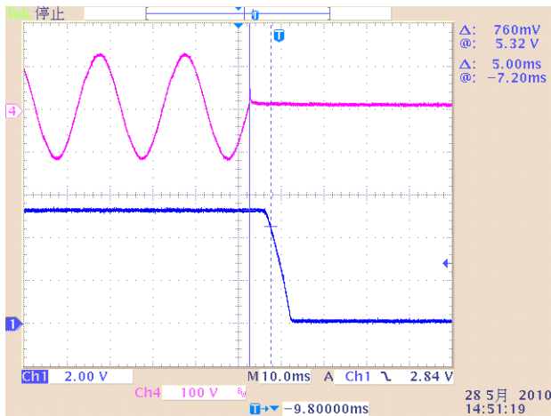
图 5 90V 关机保持时间波形
