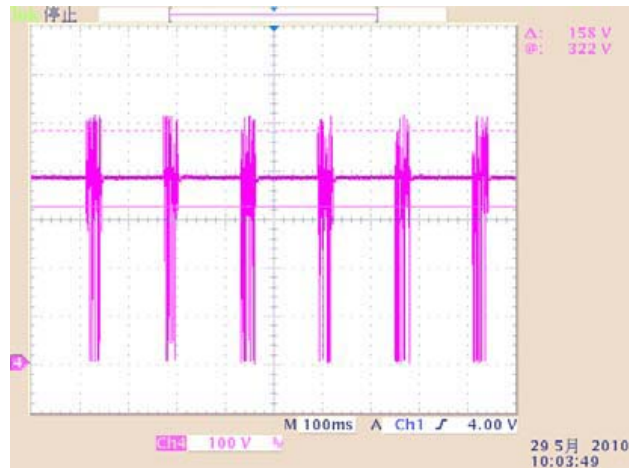
图 12 265V Voc 波形 输出短路
