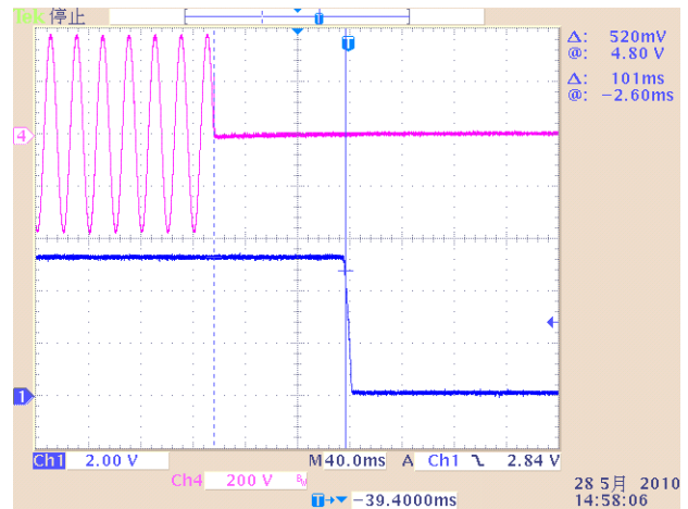
图 6 264V 关机保持时间波形
