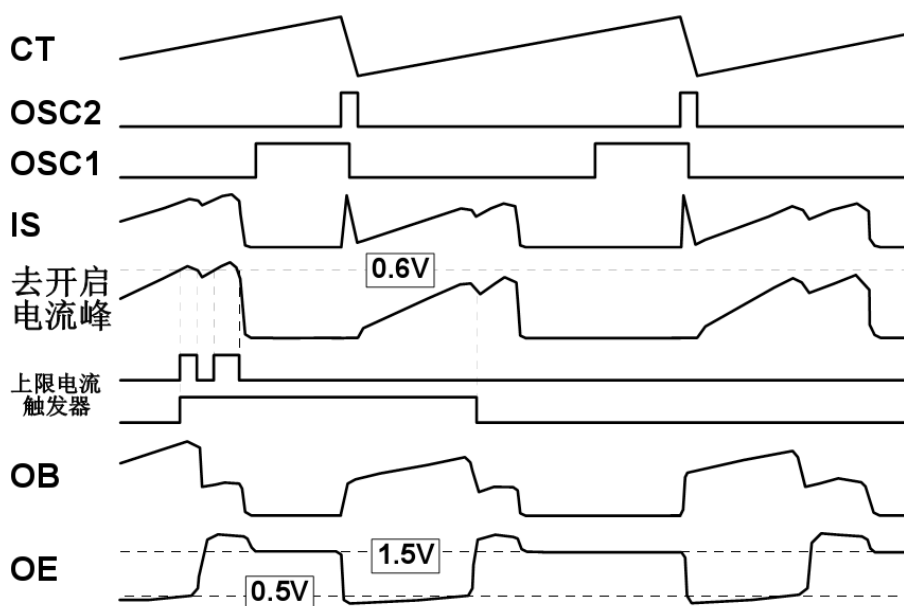
图 1 正常工作波形示意图
