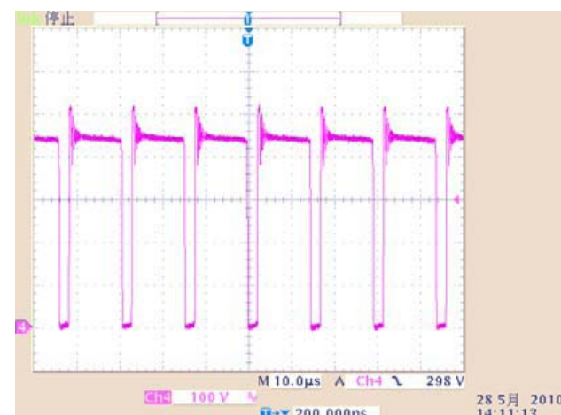
图 10 265V Voc 波形 I_o=1A
