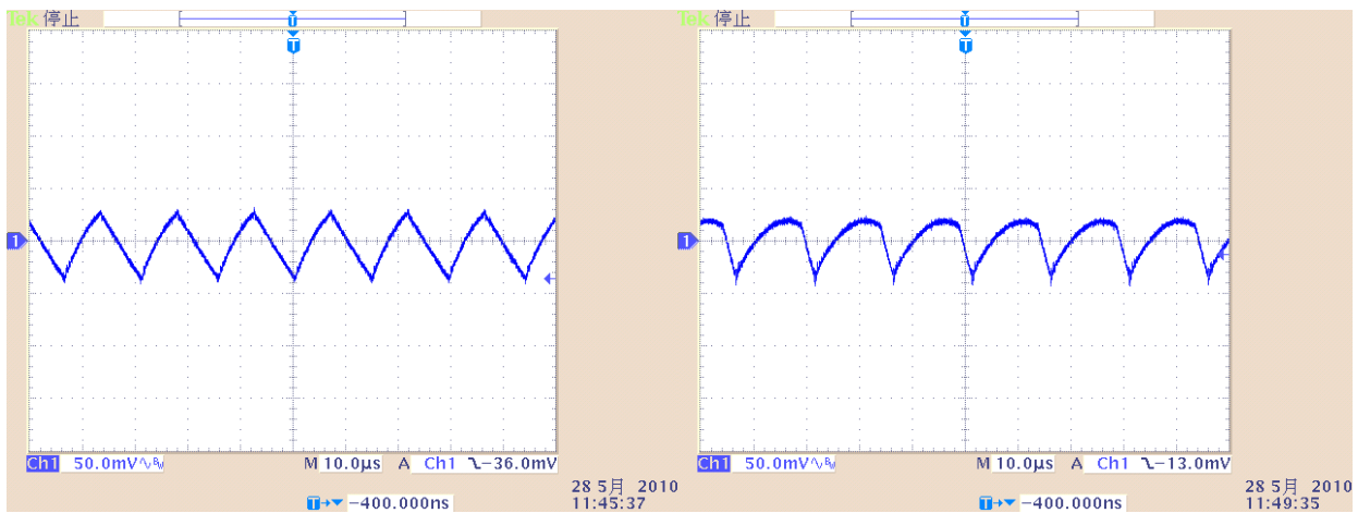
图1 输出电压纹波波形
