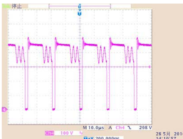
图 9 265V Voc 波形 I_o=0.5A
