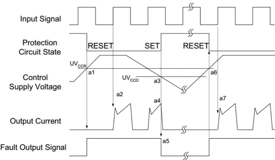
图7. 欠压保护（低端） Figure7. Undervoltage Protection (Low-side)
