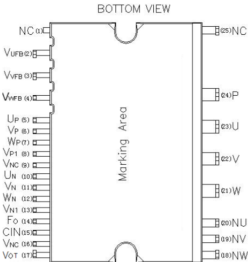
图3. 引脚布局（仰视图） Figure3. Pin Configuration (Bottom View)
