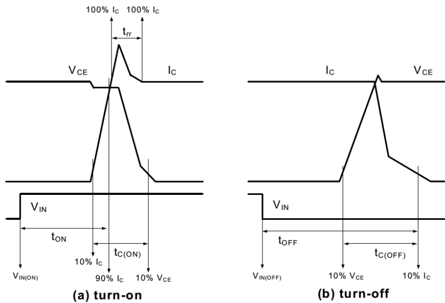
图6. 开关时间定义 Figure6. Switching Time Definition
