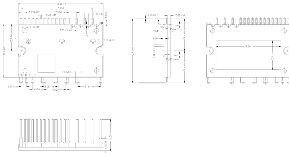
图15. 封装轮廓
