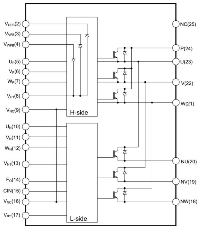
图4. 引脚布局和内部框图（仰视图） Figure4. Pin Configuration and Internal Block Diagram (Bottom View)
