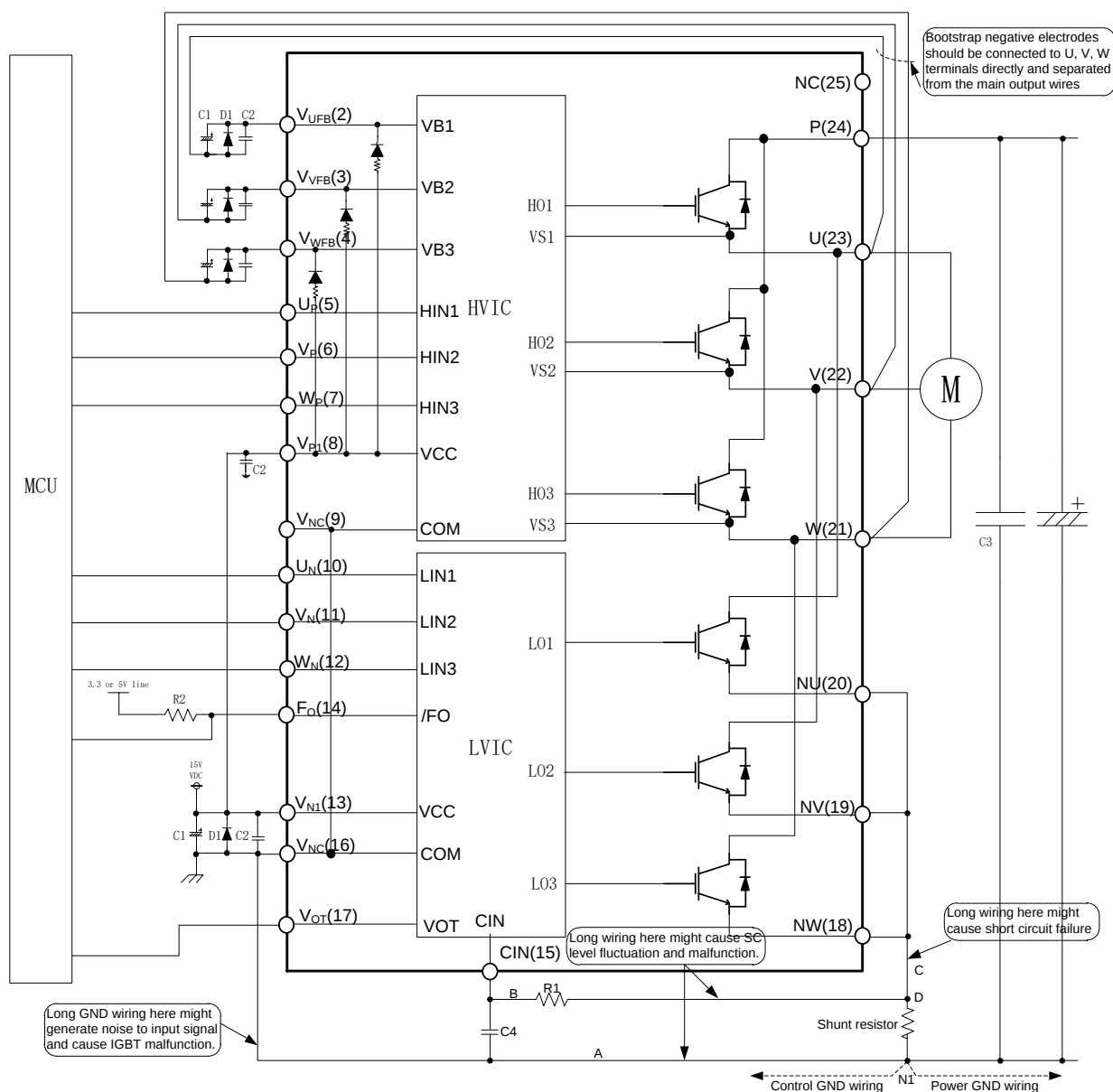
图13. 典型应用电路
