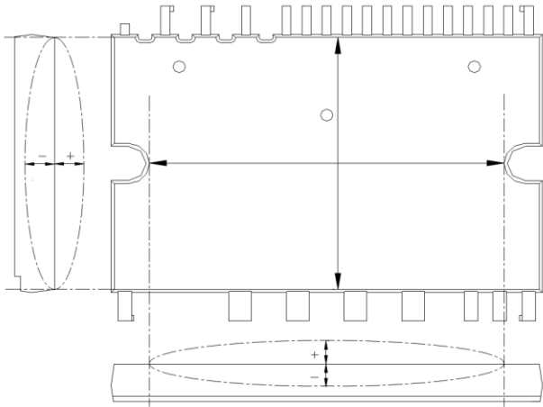
图5. 平面度测量位置 Figure5. Flatness Measurement Position
