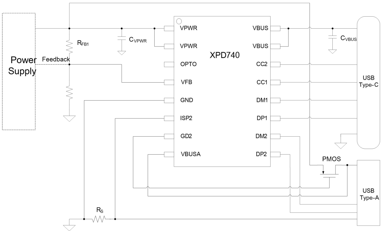
DC-DC 应用图
