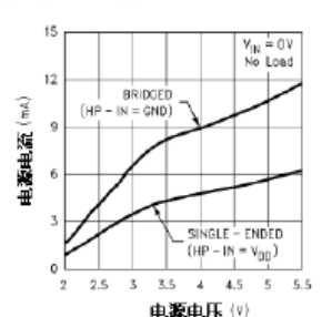
电源电流 vs 电源电压
