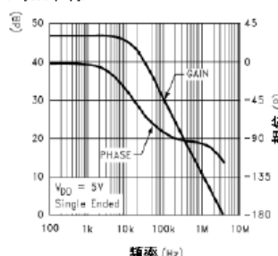
开环频率响应
