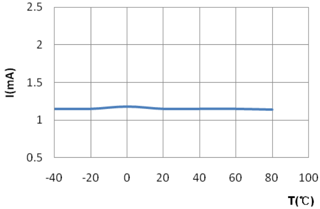
Vdd(V)=2.7V , Isopavg—TA
