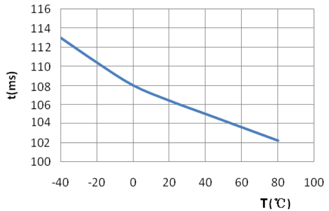
Vdd=2.7V, tstb—TA
