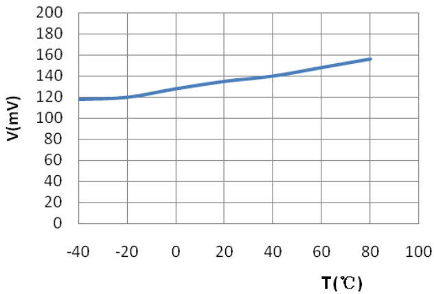
Iout=1mA , VQSAT—TA
