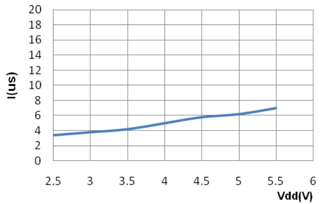
TA=20°C, Isstb—Vdd
