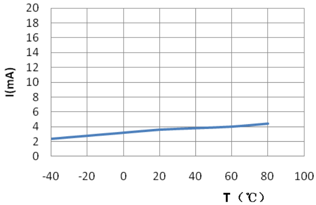
Vdd=2.7V, Isstb—TA
