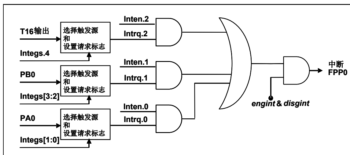
图 6: 中断硬件框图
