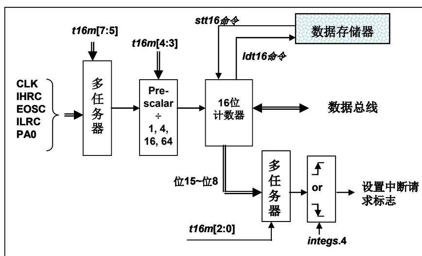
图 4: Timer16 模块框图
