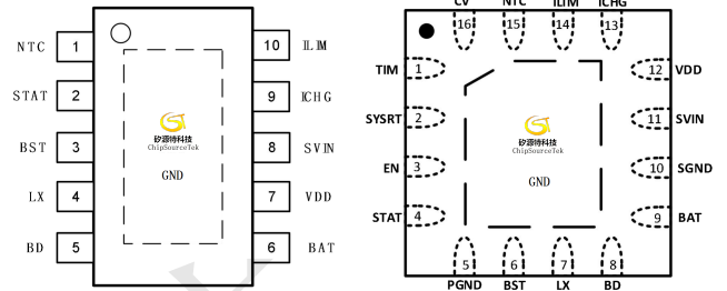
图 3. 引脚排列
