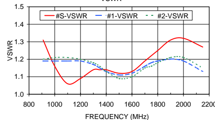
ZAPD-2-22-75+ VSWR
