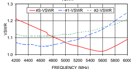
ZAPD-50W VSWR
