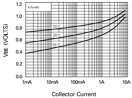
V_{BE(sat)} vs I_C
