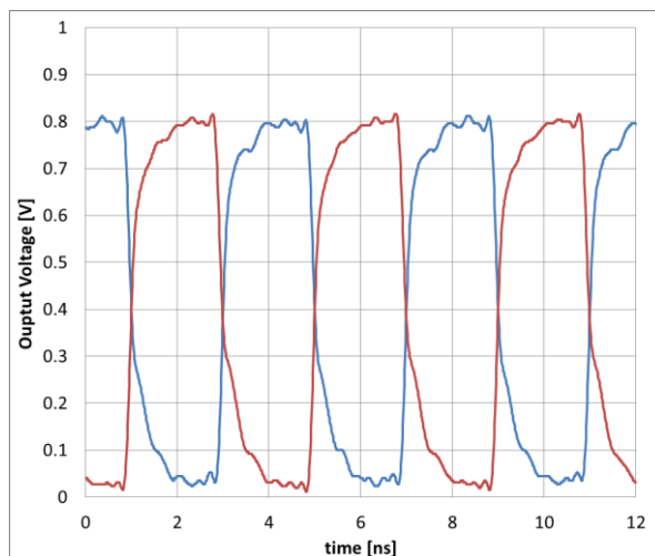
Figure 20. 250MHz HCSL
