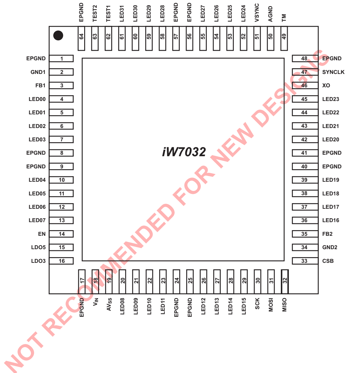
Figure 4.1 : iW7032 Pin Configuration
