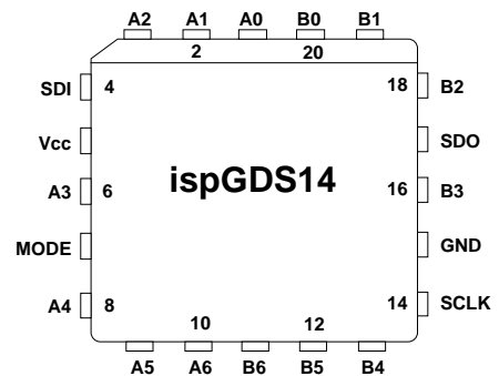
20-Pin PLCC
