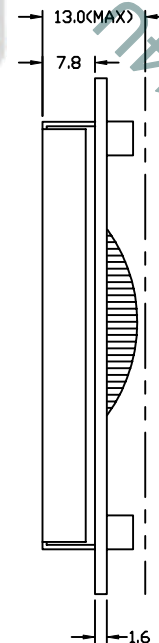
DETAIL: A
