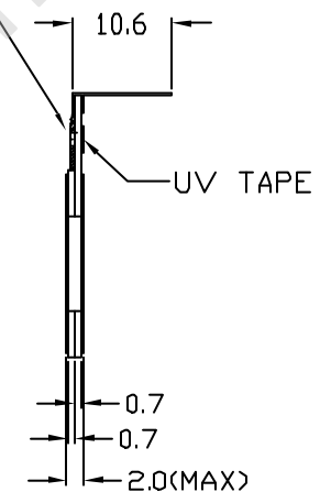
DETAIL A:
