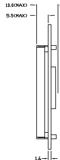
DETAIL A:
