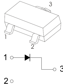
SOT-23
