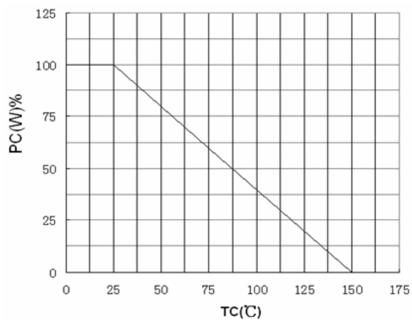
P_C - T_C
