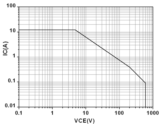
SOA
