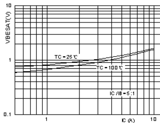
V_{BE}(\text{sat}) - I_C
