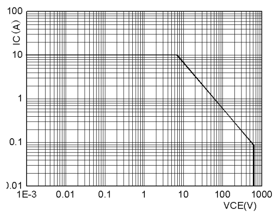
SOA
