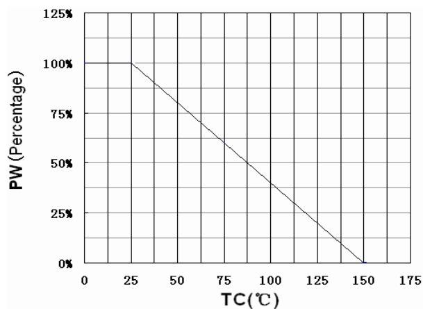
P_C - T_C
