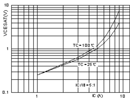
V_{CE}(\text{sat}) - I_C
