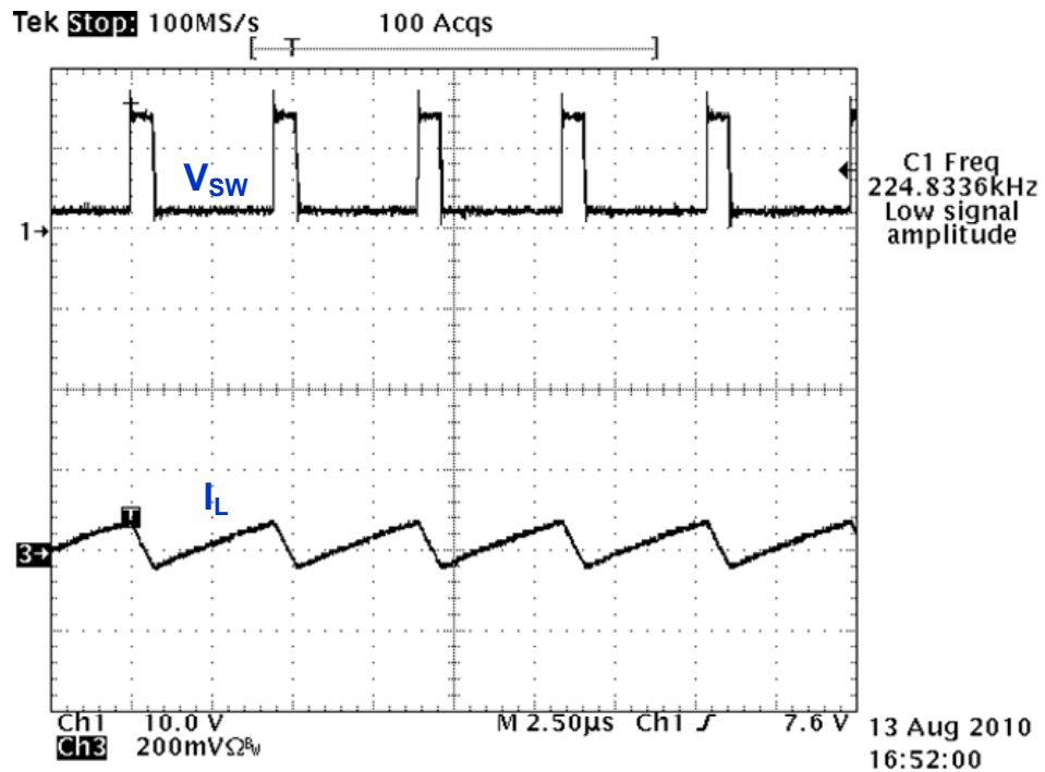
Switching waveform ( V_{IN}=12V 、 R_{SEN}=0.27\Omega 、3-LED)
