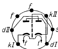
Sockelschaltschema
