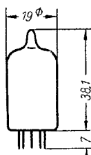
max. Abmessungen
