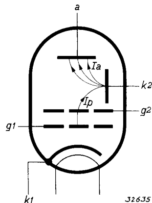
Abb. 3 Schematische Darstellung des Elektrodensystemes der Sekundäremissionsröhre. Die Primärelektronen, die die Kathode k_1 verlassen, werden auf die Sekundäremissionskathode k_2 gelenkt. Die hieraus ausgelösten Sekundärelektronen wandern zur Anode. Die Pfeilrichtung gibt die Bewegung der Elektronen an und ist dem konventionellen Strom entgegengesetzt.
