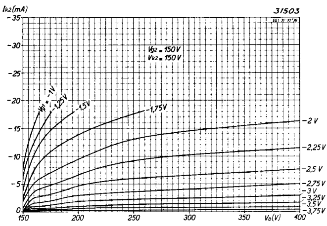
Abb. 10 Strom von der Sekundäremissionskathode als Funktion der Anodenspannung bei verschiedenen negativen Gitterspannungen.
