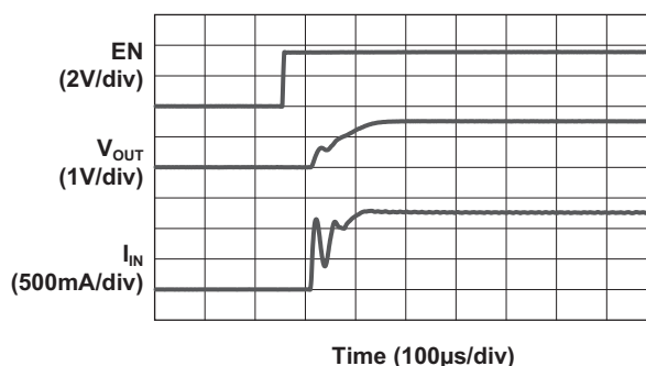
Enable Soft Start
