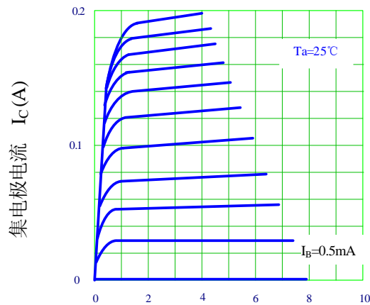
I_C - V_{CE} 特性 (典型)
