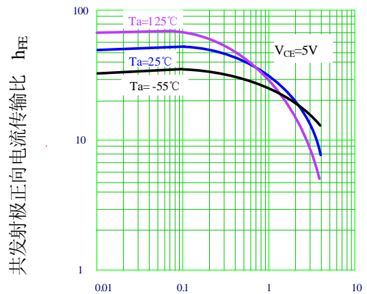
h_{FE} - I_C 温度特性 (典型)
