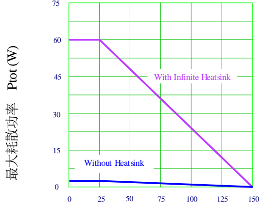
P_{tot} - T_a 关系曲线
