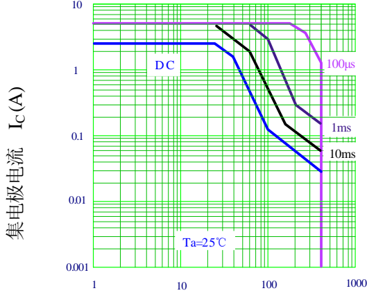
安全工作区 (单脉冲)
